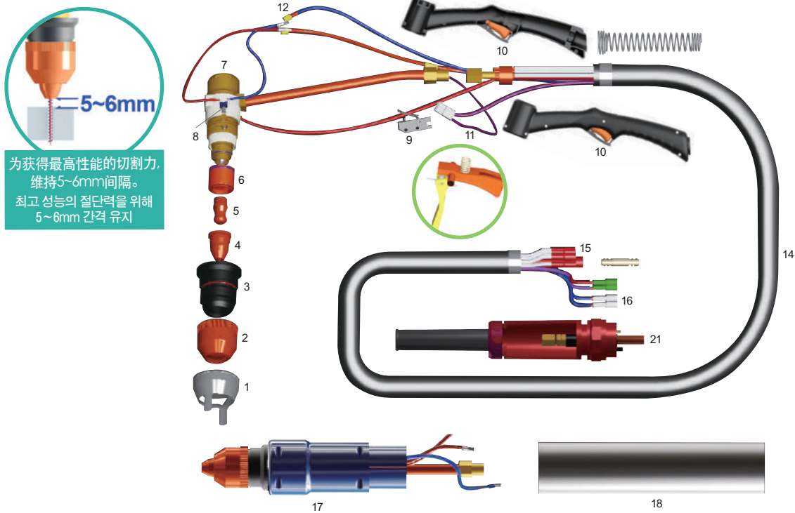
WTPX125A 配件名称 신기전 무고주파 플라즈마 절단 부품명칭
