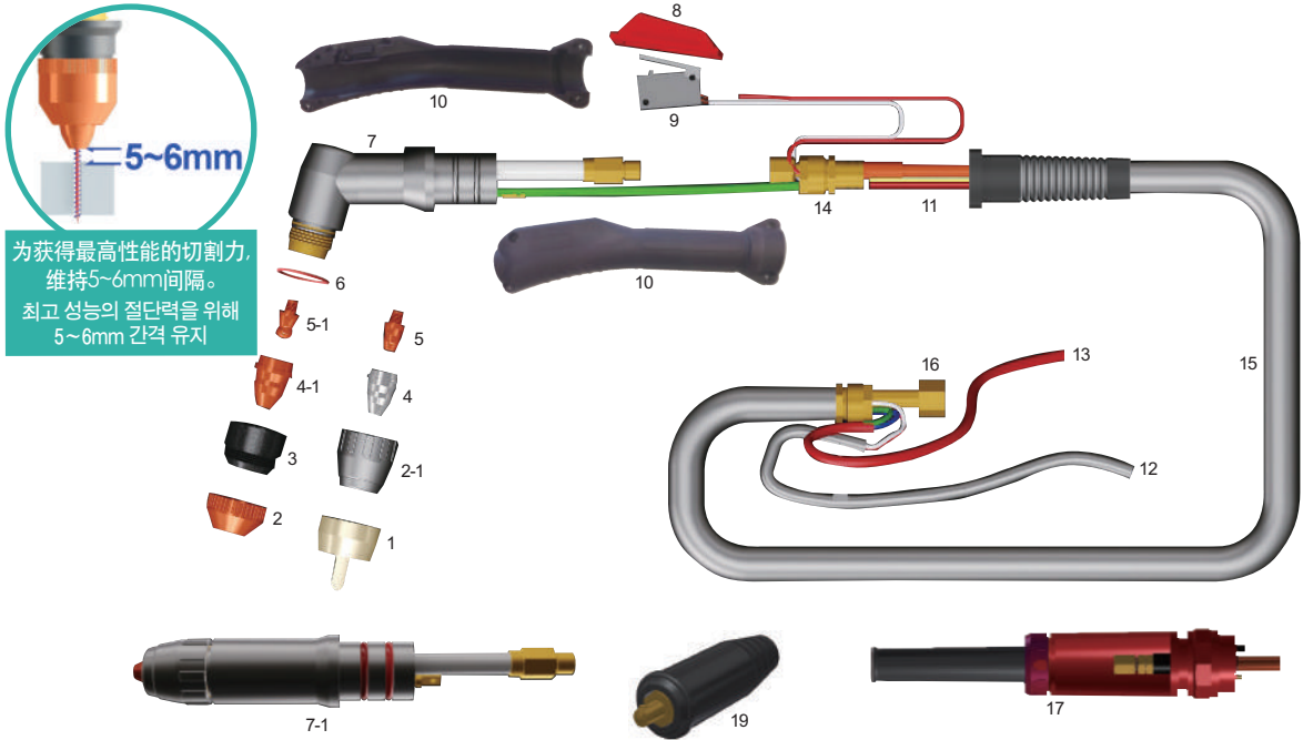
WTP60A 配件名称 신기전 프라즈마 절단 부품명칭
