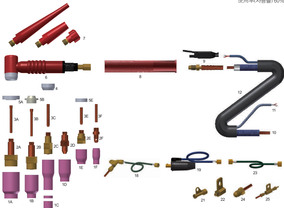
WT17 空冷一体配件名称 / WT17 원피스 공냉 부품 명칭
