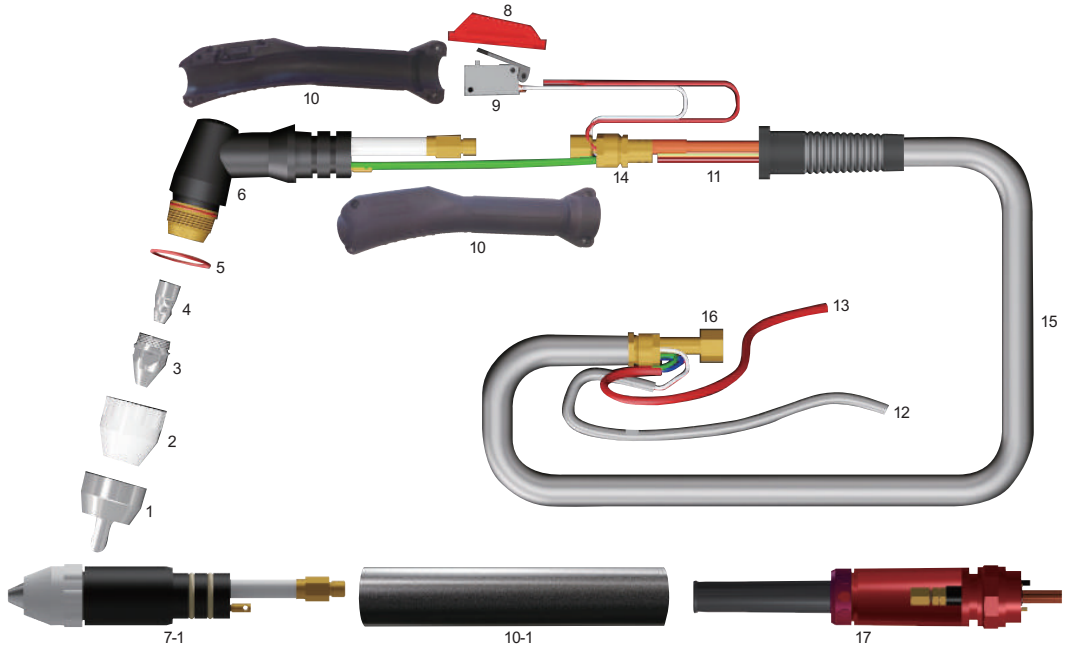
WTP80A 配件名称 파나소닉 프라즈마 절단 부품명칭
