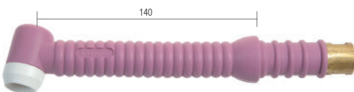
WON350A 空冷可弯曲长焊枪 WT26FLL 6-83 WON350A 公냉 후렉시블 롱 토치 WT26FLL 6-83
