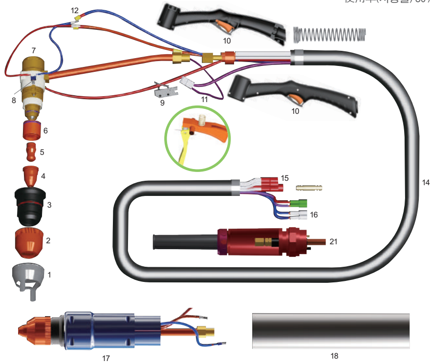
WTPX105A 配件名称 신기전 무고주파 프라즈마 절단 부품명칭
