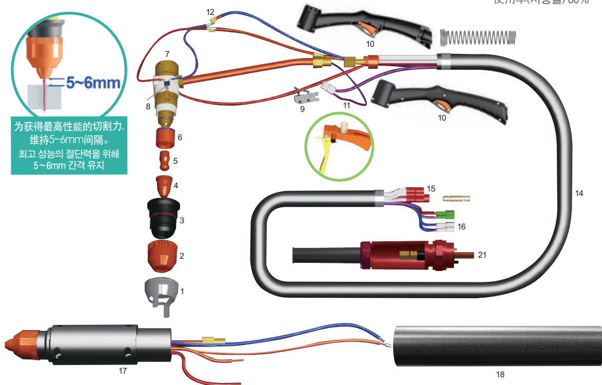
WTPX65A 配件名称 신기전 무고주파 프라즈마 절단 부품명칭
