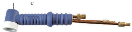
WON500A 特制水冷可弯曲焊枪 WT500FW 40-104-3 WON500A 수냉 특수 후렉시블 토치 WT500FW 40-104-3
