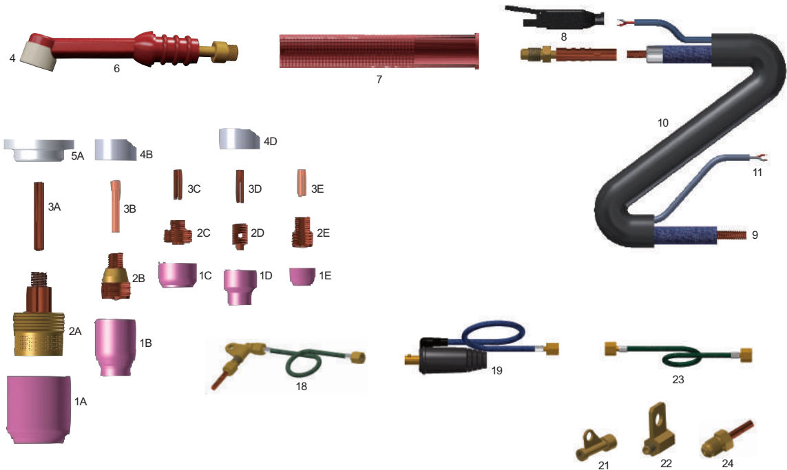
WT24 空冷一体配件名称 / WT24 공냉 원피스 부품 명칭
