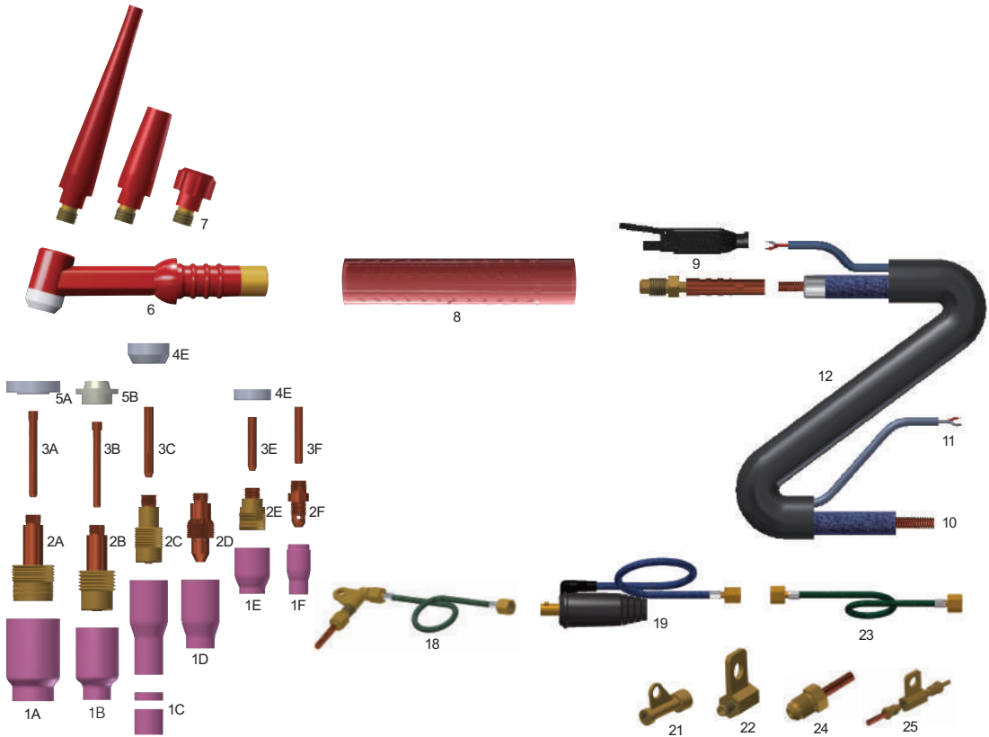
WT26&200A 空冷一体焊枪配件名称 / WT26&200A 원피스 공냉 부품 명칭
