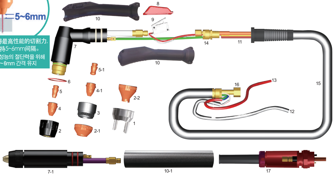
WTP120A 配件名称 신기전 플라즈마 절단 부품명칭
