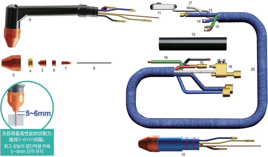
WTP100-150A 配件名称 신기전 수냉 프라즈마 절단 부품명칭
