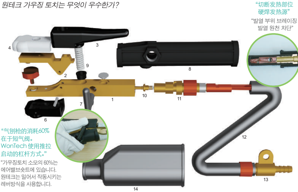
800 配件名称 가우징 토치 부품명칭
