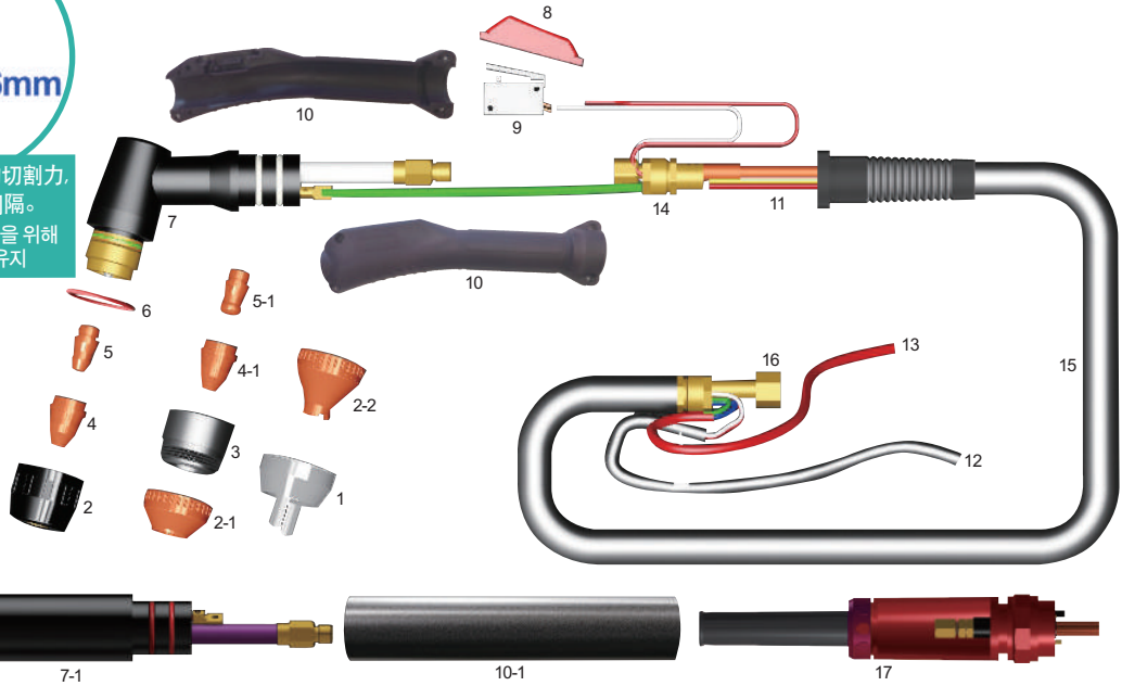
WTP100A 配件名称 신기전 프라즈마 절단 부품명칭
