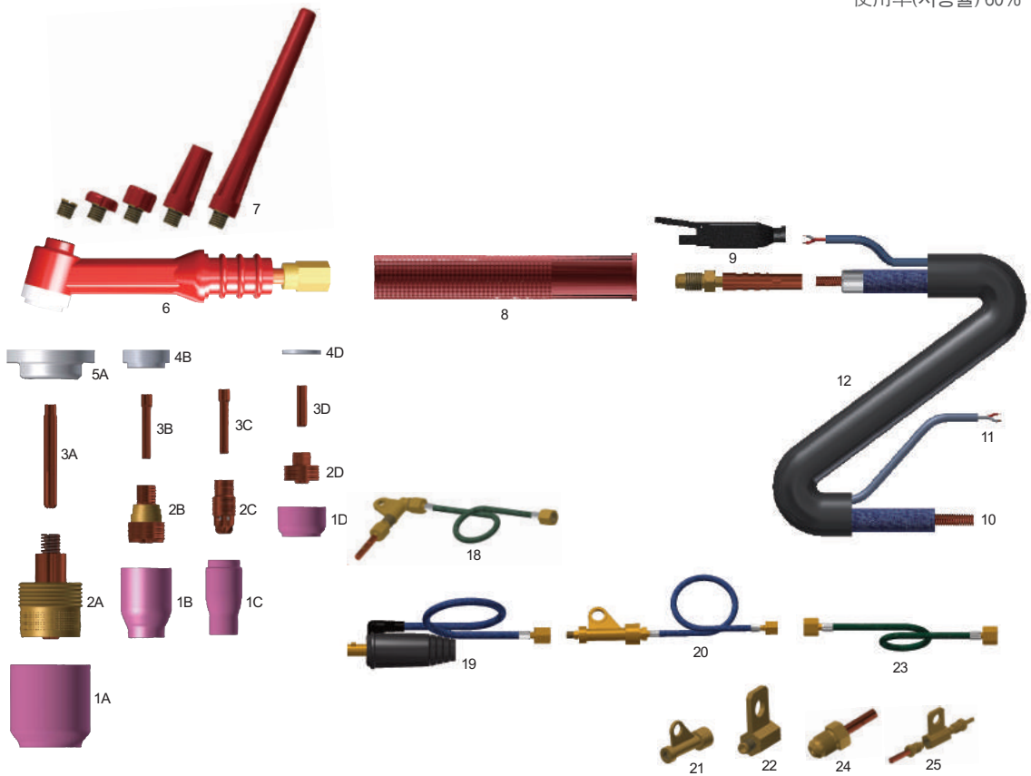
WT9 空冷一体配件名称 / WT9 공냉원피스 부품 명칭
