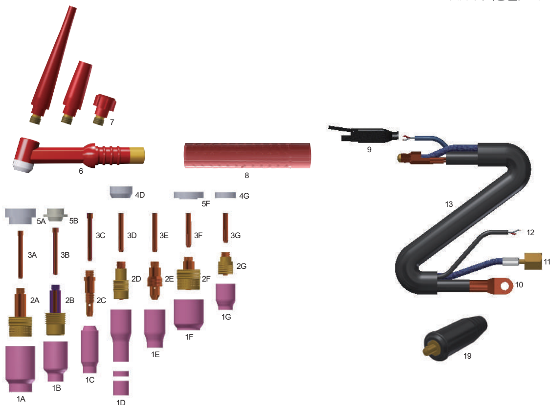
WT26&200A 空冷两件焊枪配件名称 / WT26&200A 투피스 공냉 부품 명칭
