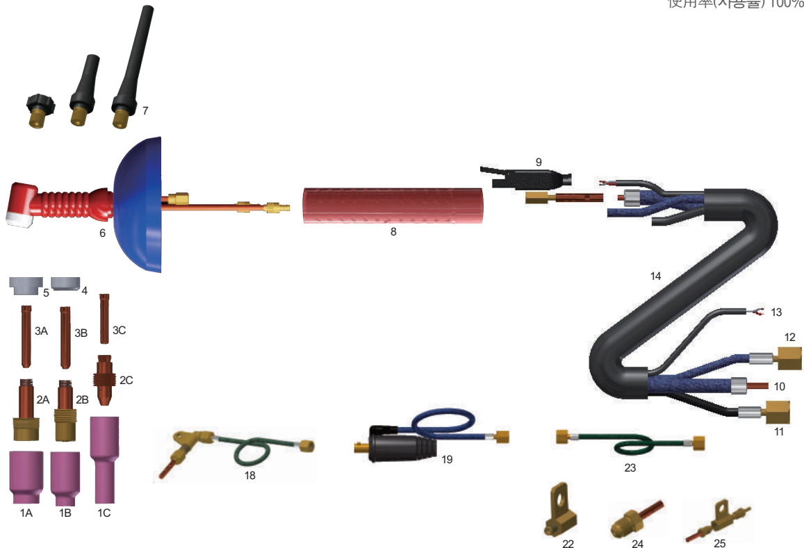
WT40&400A 大容量水冷焊枪组配件名称 / WT40&400A 고용량 수냉부품 명칭
