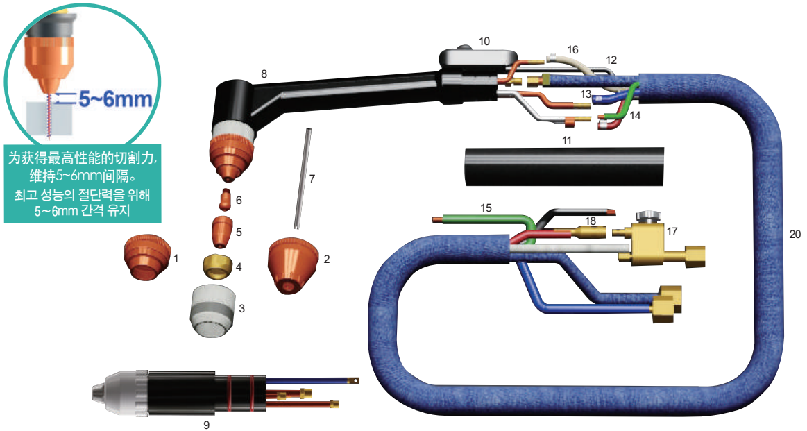
WTP100-180A 配件名称 신기전 수냉 프라즈마 절단 부품명칭
