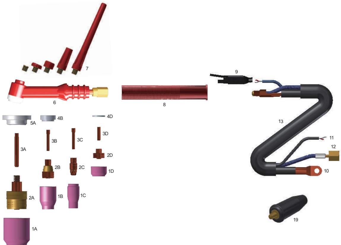
WT9 空冷两件焊枪的配件名称 / WT9 공냉투피스 부품 명칭
