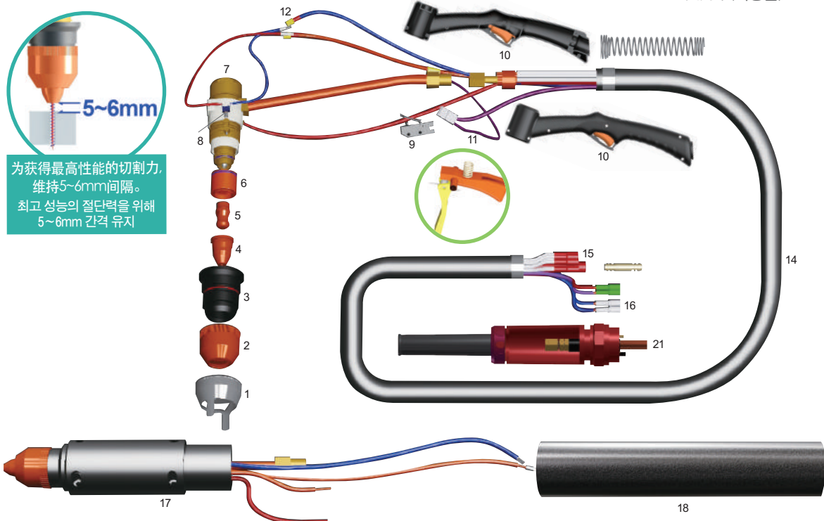
WTPX85A 配件名称 신기전 무고주파 프라스마 절단 부품명칭
